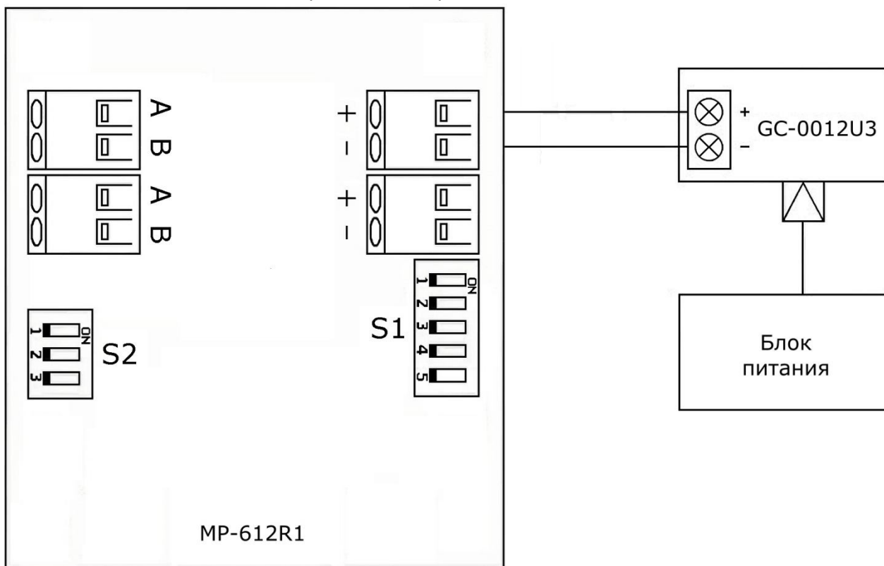
Рисунок 6.1. Схема соединений комплекта MP-922W7
