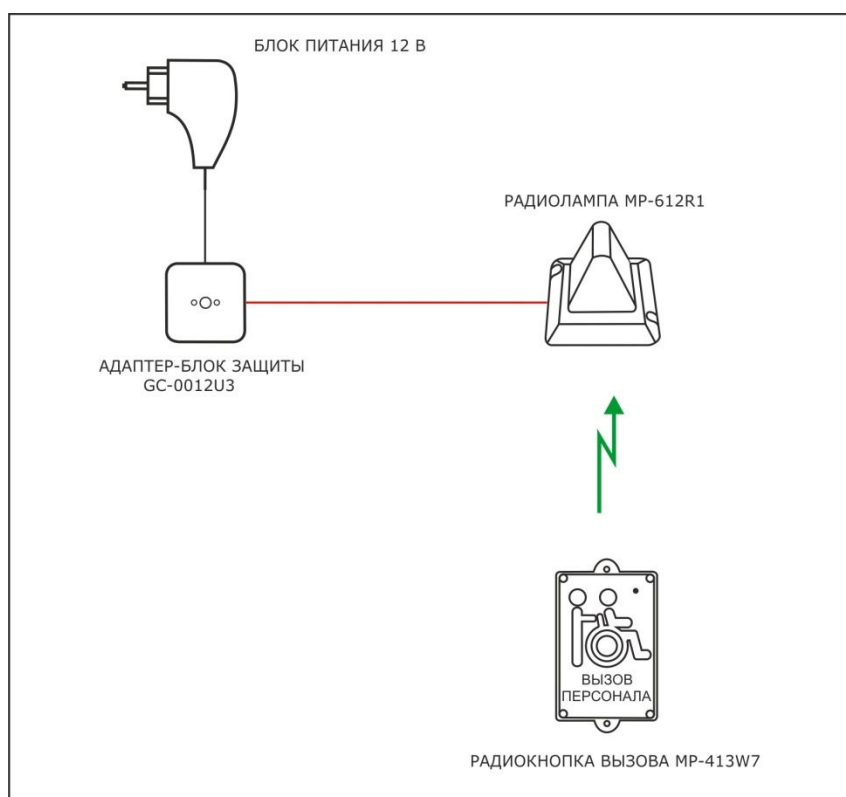
Рисунок 2.1. Структурная схема комплекта MP-922W7
